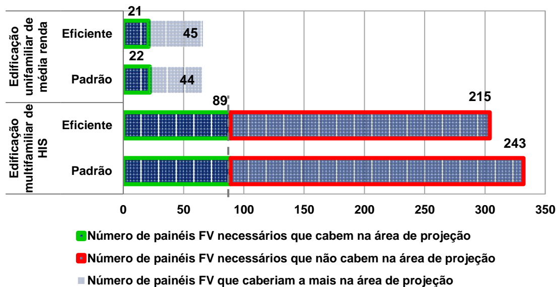
Figura 64 – Número de painéis fotovoltaicos para Net-Zero: arquétipos do setor residencial Fonte: elaboração própria
