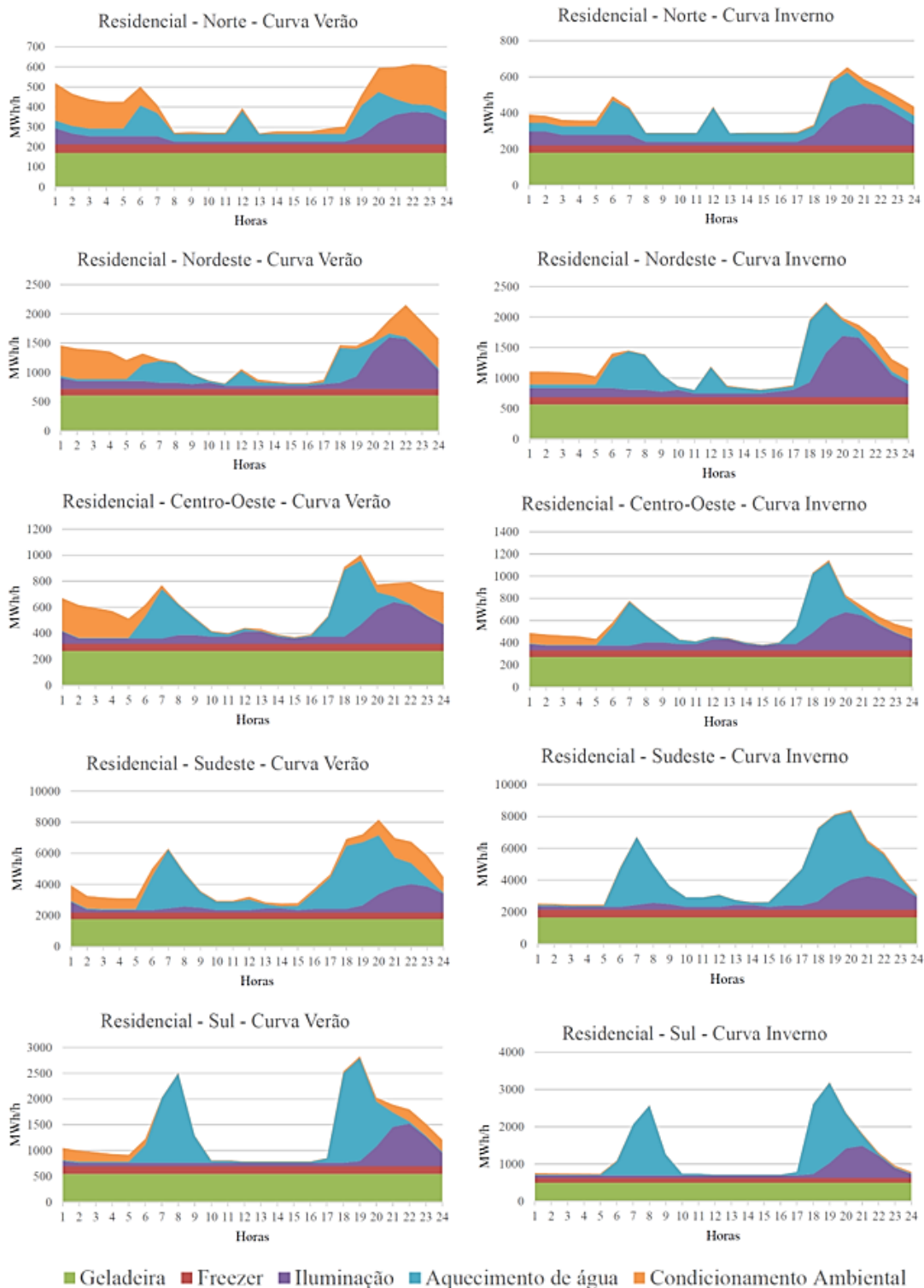
Figura 43 – Curvas de carga residenciais para as diferentes regiões brasileiras, no verão e no inverno Fonte: VIEIRA (2016)
