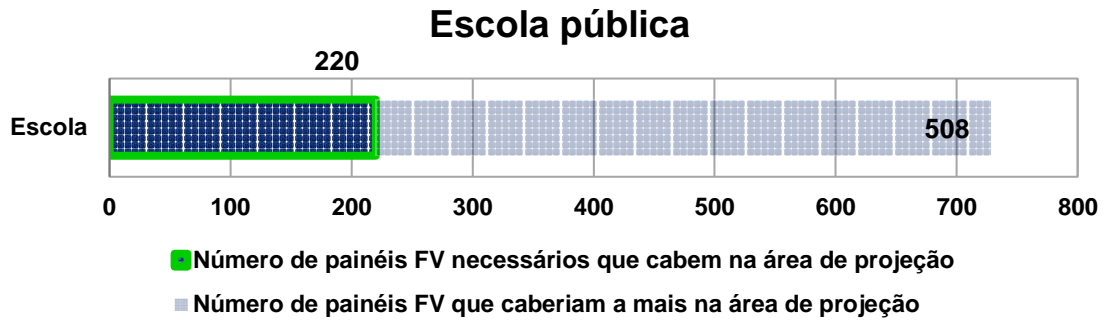
Figura 65 – Número de painéis fotovoltaicos para Net-Zero: arquétipo escola Fonte: elaboração própria
