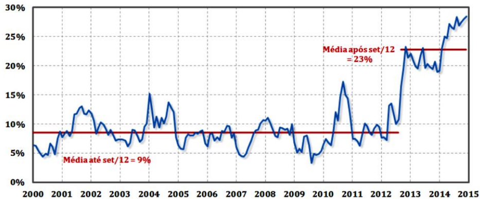
Figura 17 – Participação da Geração Térmica no Total da Carga do SIN (%) Fonte: ROMEIRO et al (2015)
