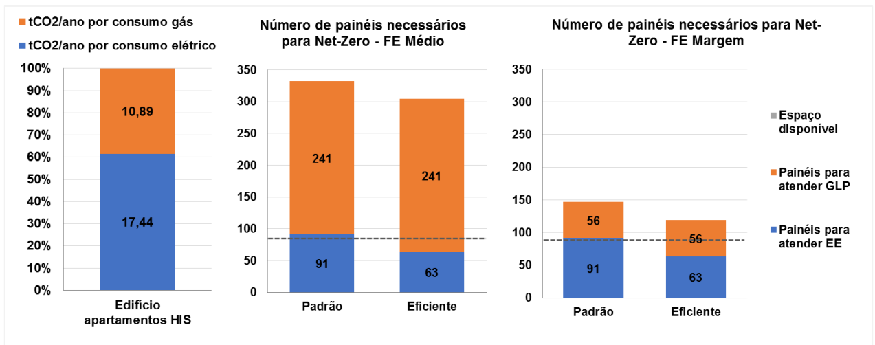
Figura 69 – Comparação entre o uso do fator médio e fator na margem de operação, edificação multifamiliar de HIS Fonte: elaboração própria
