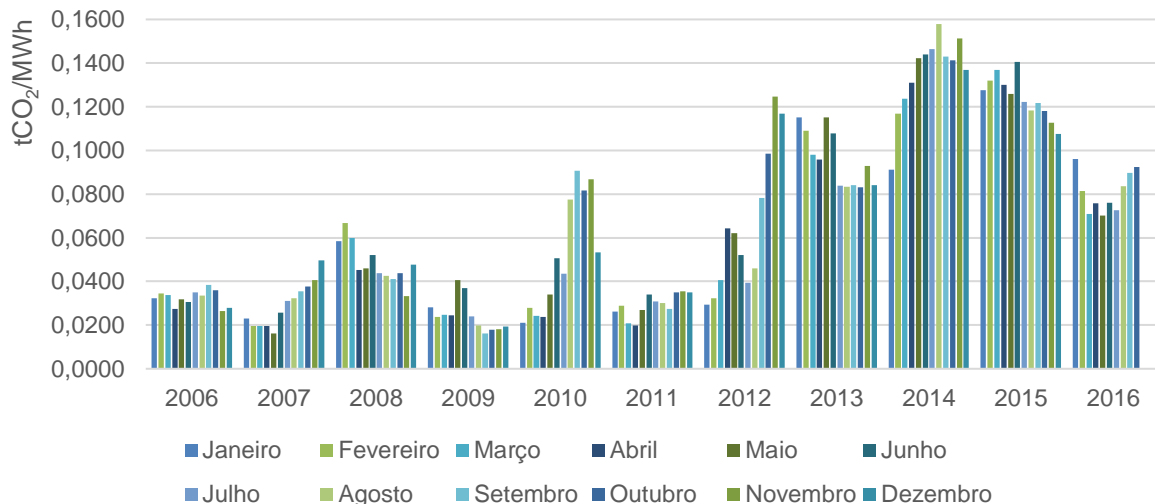
Figura 16 – Fatores de emissão médio mensais em tCO 2 /MWh, de 2006 a 2016 Fonte: elaboração própria, com dados do MCTI (2017)
